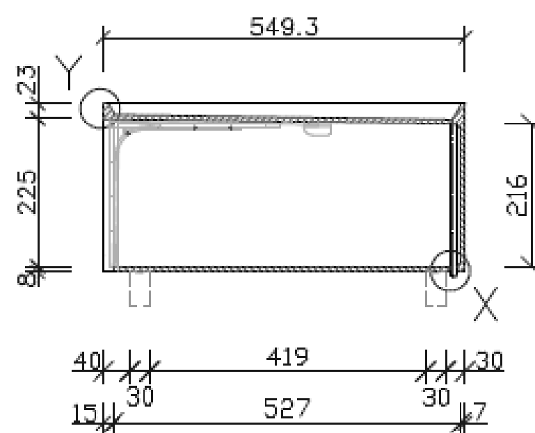
Langsdoorsnede
