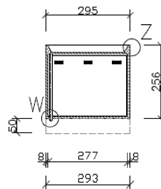
Dwarsdoorsnede
